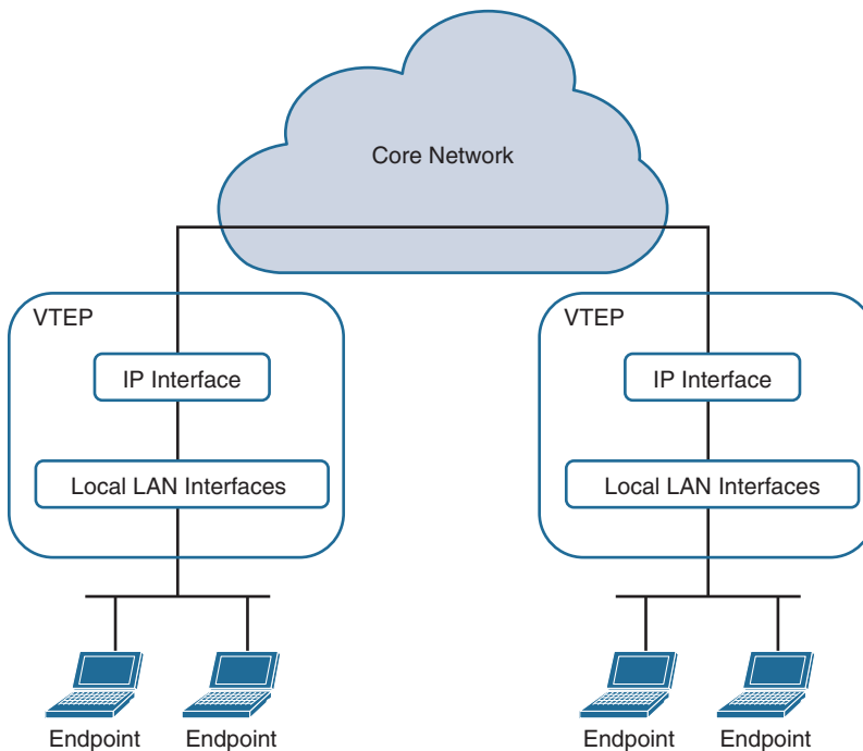
Figure 16-14 VXLAN VTEP
